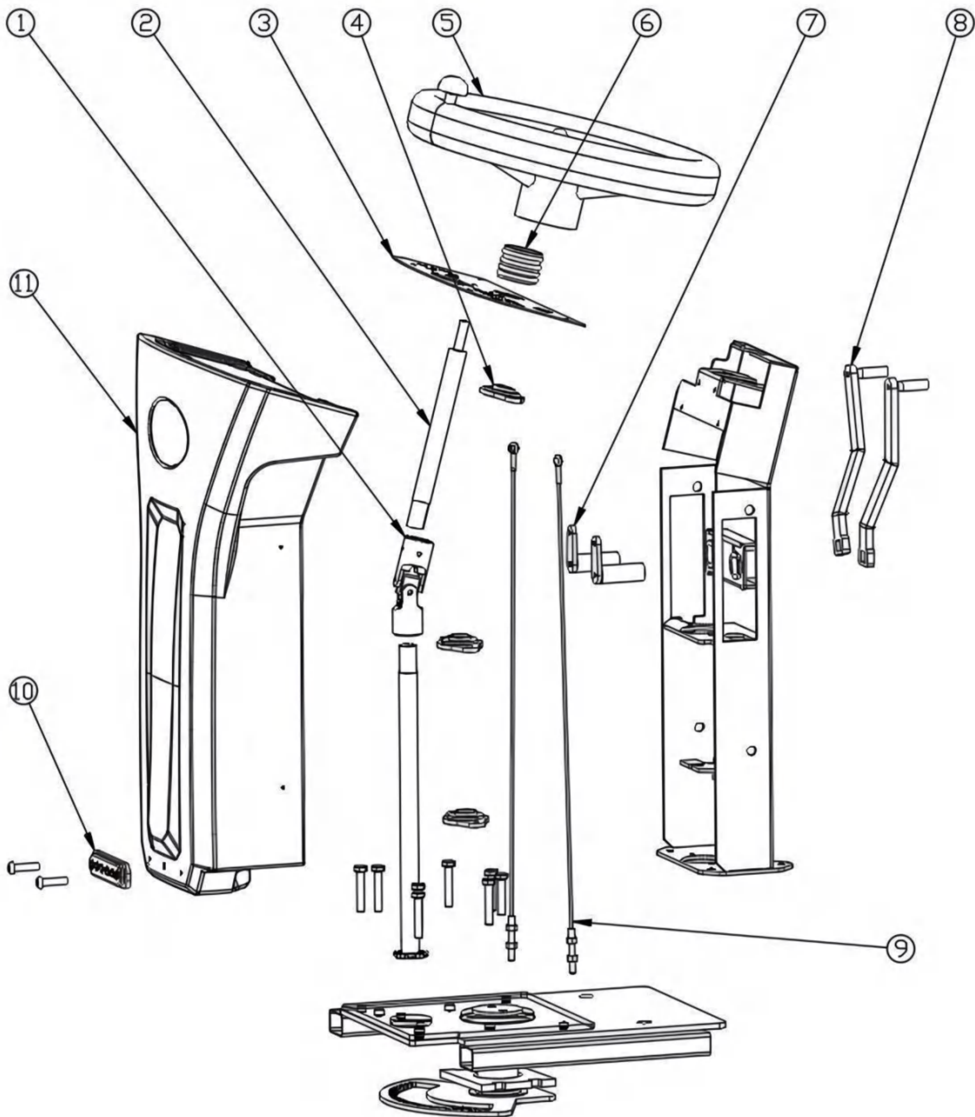
Fig. 3 -Steering Group
